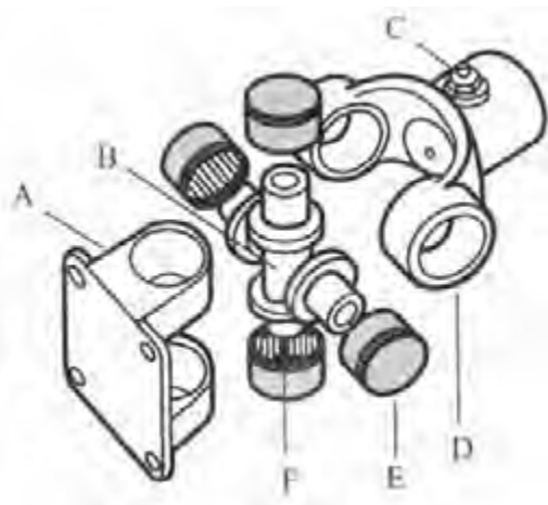
شکل ۲۹۲- مجموعه‌ی قطعات چهار شاخه‌ی گاردان
