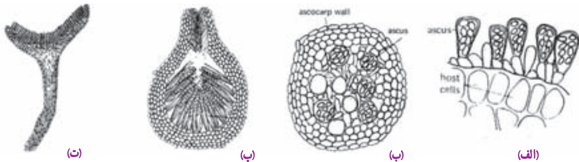
الف) ژیموتشیوم (ب) کلیستوتشیوم (ب) پری تشیوم (ت) آپوتشیوم شکل ۴-۴ رده بندی آسکومایکوتینا بر اساس نوع آسکوکارپ
