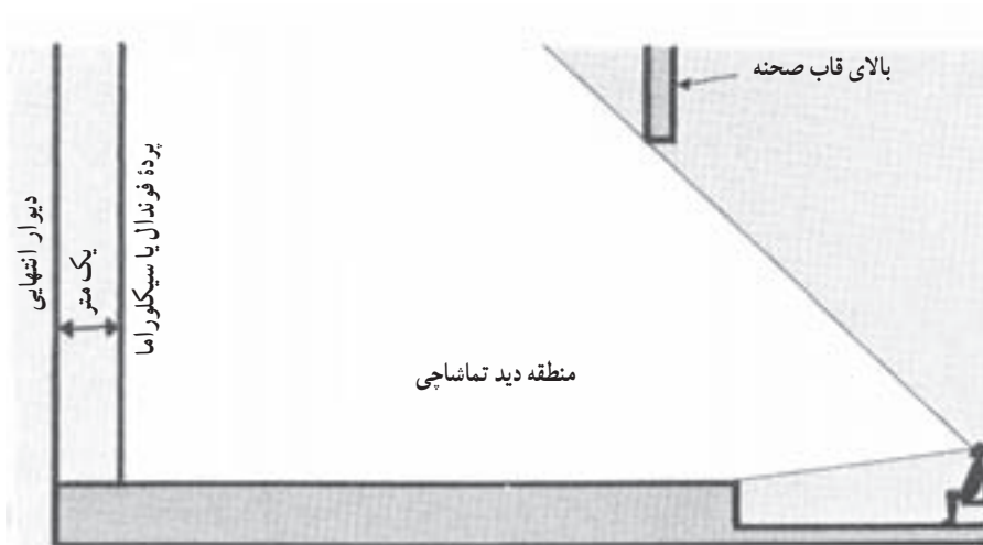
▲ شکل ۷-۵- برش یک صحنه و پائین‌ترین و بالاترین خط دید
