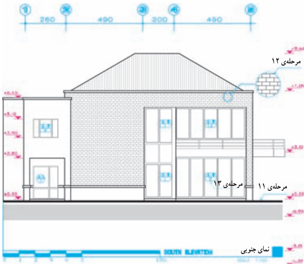
شکل ۹-۵- مراحل ترسیم نما
