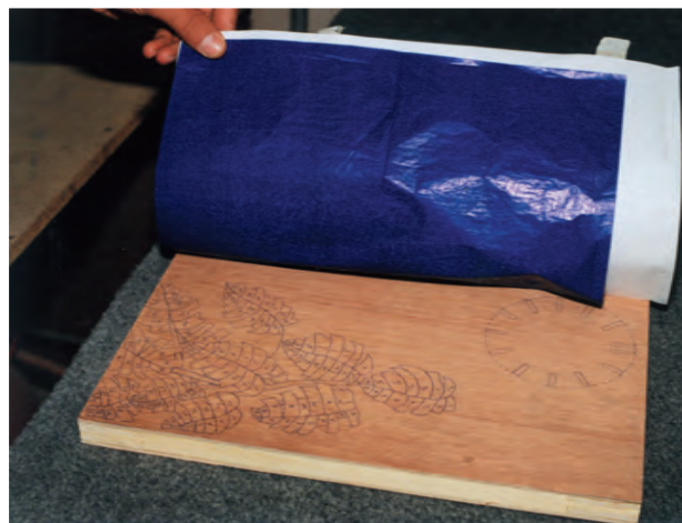
تصویر ۲-۱۱-۲- طرح به وسیله کاغذ کارین دقیقاً به روی زیر ساخت منتقل می‌شود.
