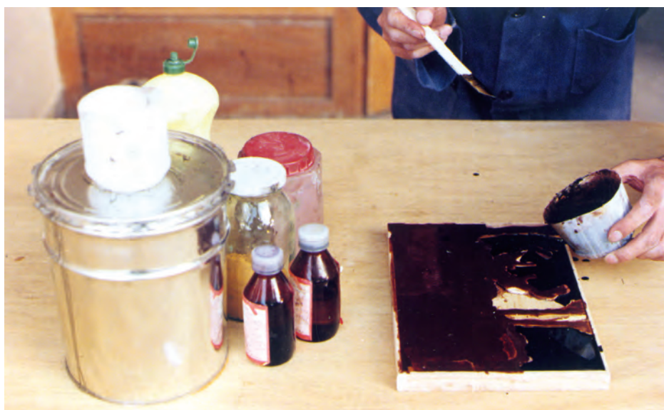
تصویر ۱۰-۱۱-۲- پلی استر بعد از مخلوط شدن با رنگ و مواد شتاب دهنده و سخت کننده روی تابلو ریخته می شود.
