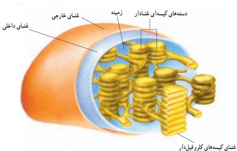
شکل ۴-۲- کلروپلاست
