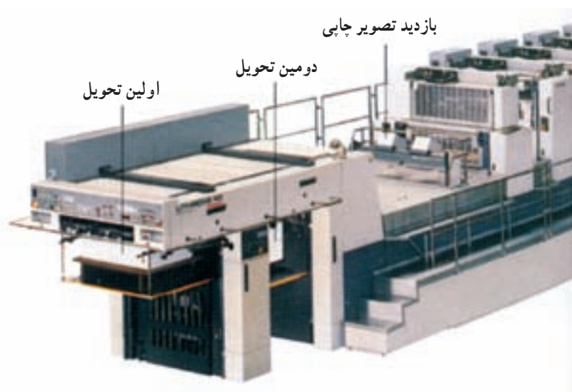
شکل ۱۱-۵- تحویل دو واحدی و سیستم بازدید تصویر چاپی
