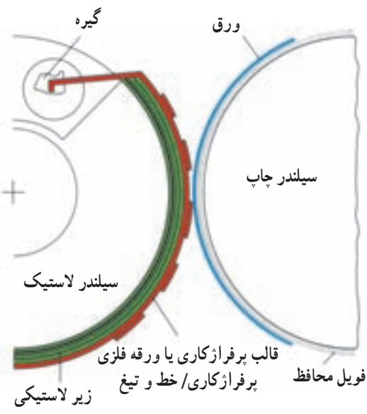
شکل ۷-۵- ورق‌های فلزی پرفراژیاری، قابل نصب روی سیلندر لاستیک با نوارهای خطزنی و پرفراژ که روی ورق چسبانده می شوند.
