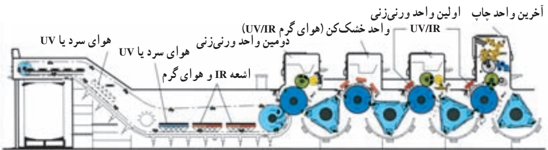
شکل ۳-۵- واحدهای ورنی زنی دوبل با واحد خشک‌کن، تحویل طولی و چندین مازول خشک‌کن
