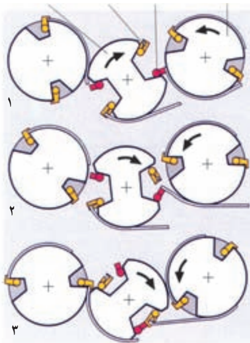
شکل ۲۶-۴- سیستم‌های برگردان ورق (سیستم تک‌درام)
