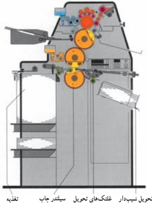
شکل ۳-۴- تحویل شیب‌دار روی ماشین چاپ کوچک تک‌رنگ افست
