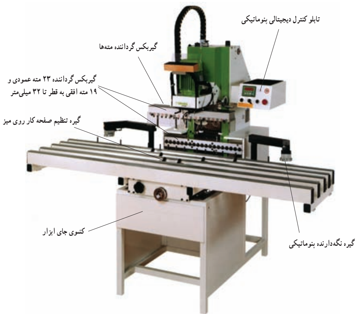
شکل ۹-۸۸- ماشین سوراخ‌زنی و لولازنی دیجیتال پنوماتیک
