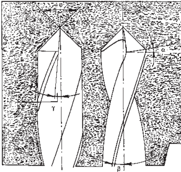
شکل ۱۱-۹- مته مناسب سوراخکاری چوب‌های بهن‌برگ و صفحات چسب‌دار
