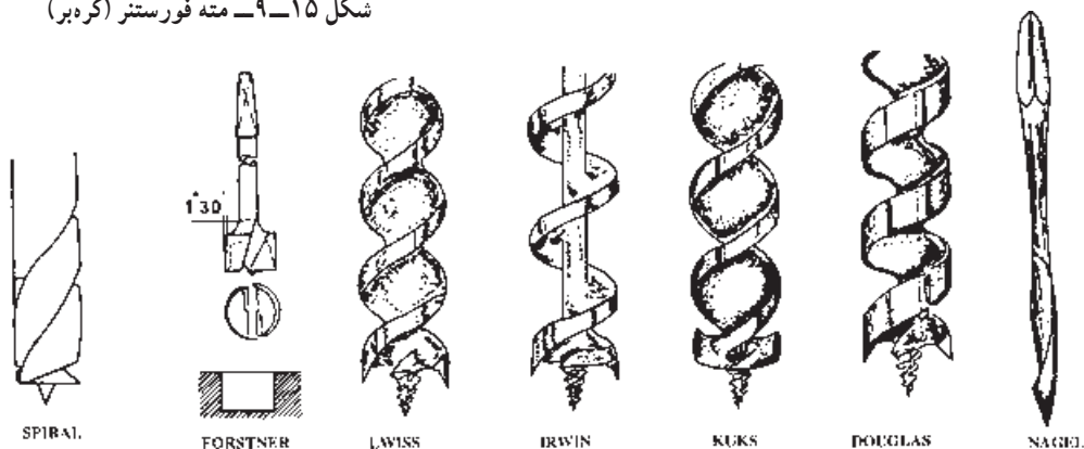
مته مدل میخی NAGEL. مته مدل داگلاس DOUGLAS. مته مدل کوکس KUKS. مته مدل ایروین IRWIN. مته مدل لویس LAWISS. مته مدل گره بر، گره زنی FORSTNER. مته مدل پیچی SPIRAL.
