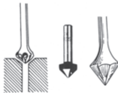
شکل ۹-۱۵/۱- مته خزینه
