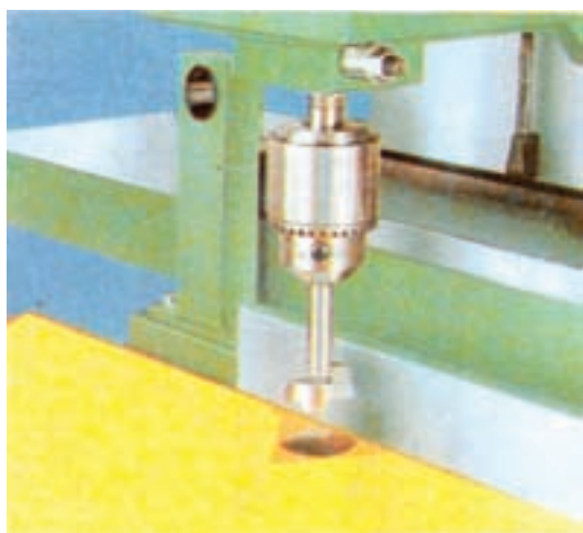
شکل ۹-۴۶- تنظیم عمق سوراخ جای لولا گازی به وسیله ماشین مته عمودی
