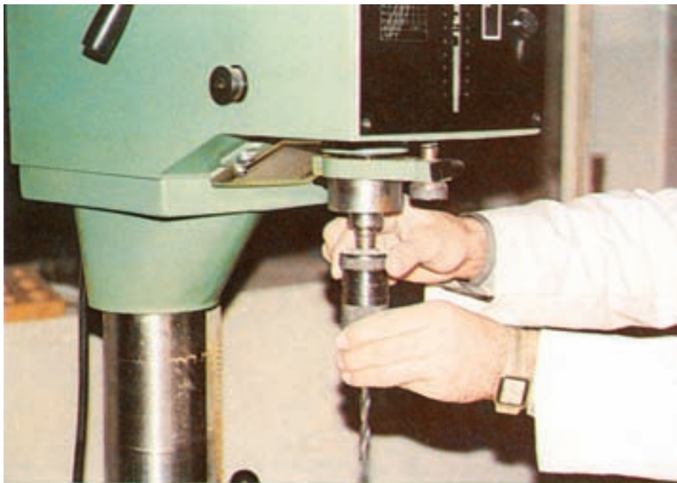
شکل ۹-۴۹- نحوه محکم کردن مته در سه نظام خودکار عمودی
