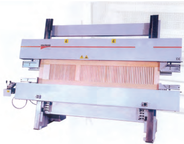
شکل ۵۶-۵- تنگ پنوماتیکی برای جمع کردن و چسباندن قاب چوبی
