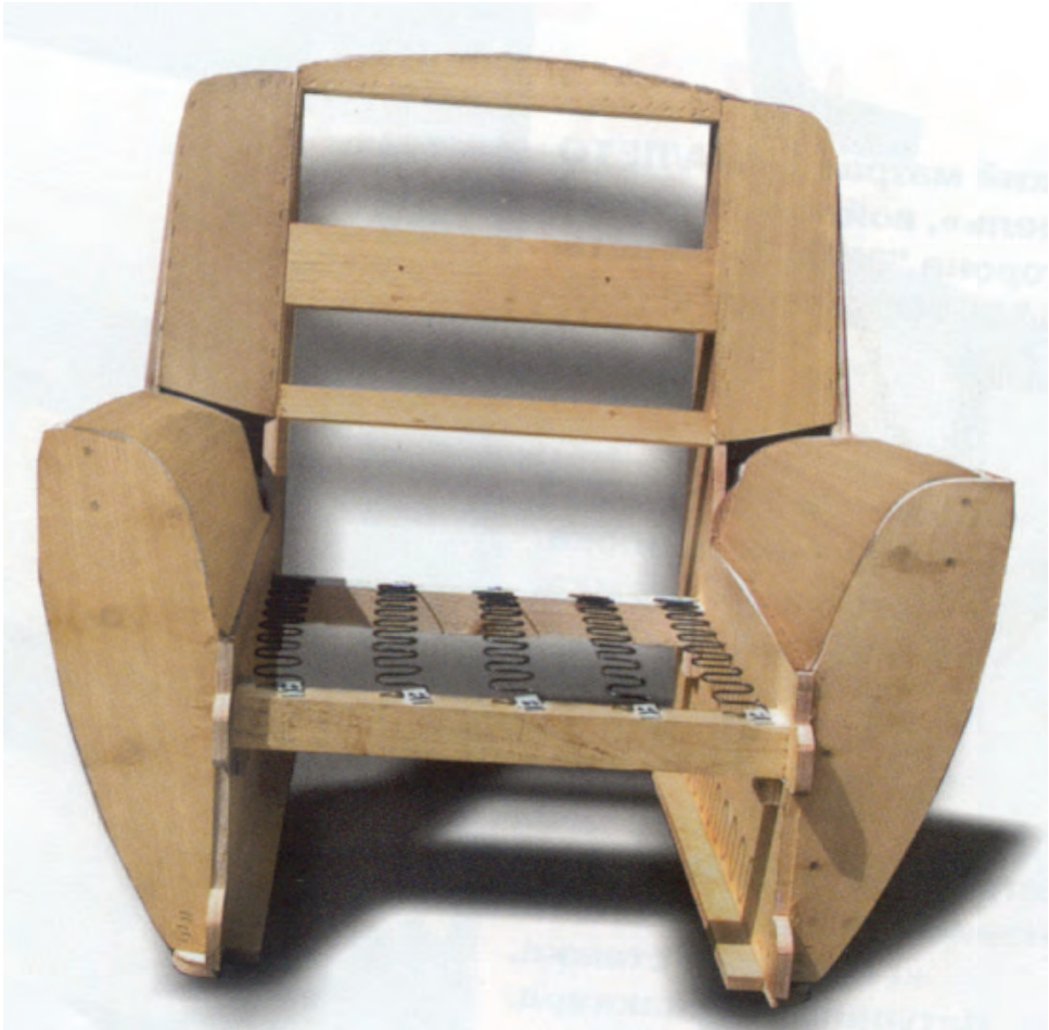
شکل ۵-۶۲- نمونه‌ی فتر کوبی کف مبیل
