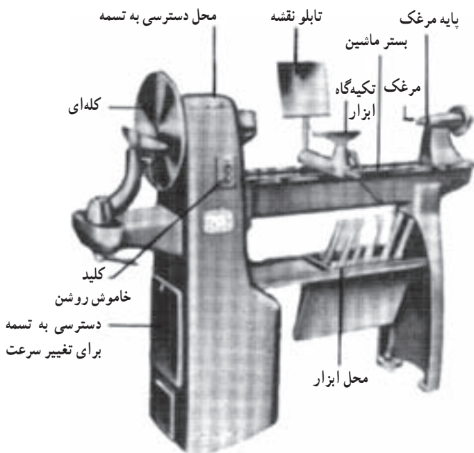
شکل ۳-۱۳- ماشین خراطی
