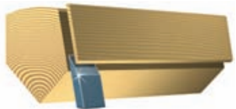
تراشه‌زنی در جهت بینابینی (به صورت عرضی)
