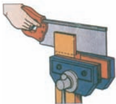
شکل ۲-۱۱- بریدن زبانه با اره‌ی پشت‌دار
