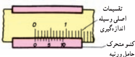
شکل ۱-۳۹- ورنیه ۰/۱ mm
