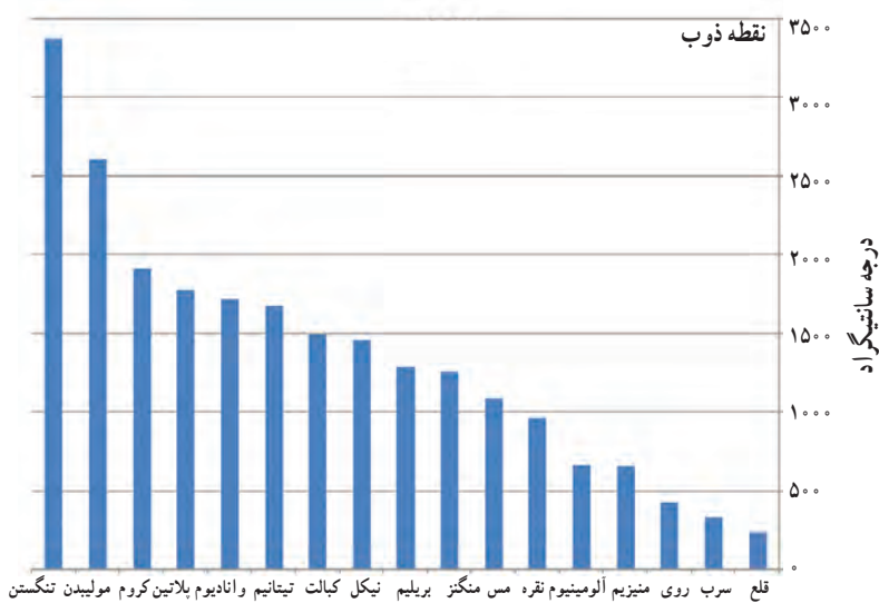
نمودار ۶-۷- مقایسه نقطه ذوب فلزات پر کاربرد در صنایع
