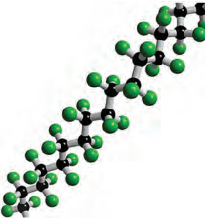
شکل ۱-۵- بخشی از یک مولکول پلیمری (تفلون)
