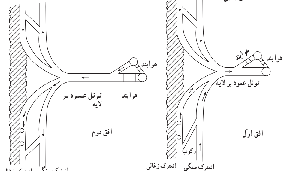
شکل ۱۳-۸- روش استخراج کارگاه بالارو و خاکریزی
