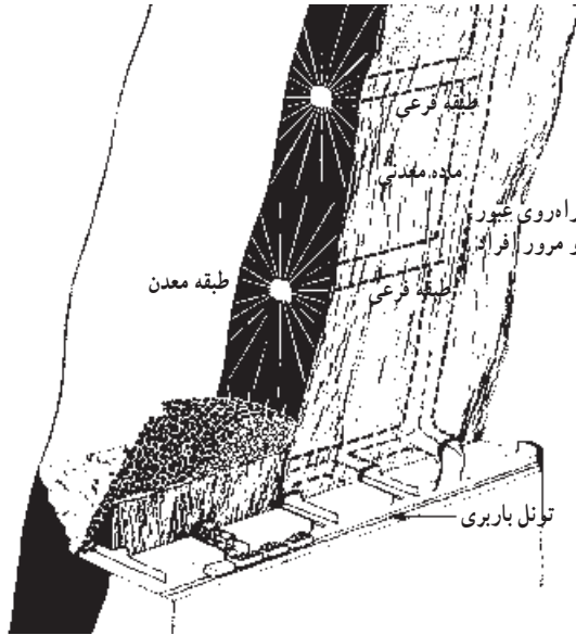
شکل ۶-۷- روش احداث طبقات فرعی
