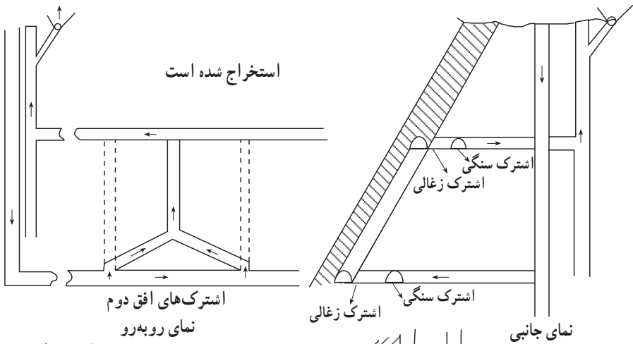
شکل ۱۲-۸- جدا کردن دوپل‌های خاکریز و زغال‌ریز
