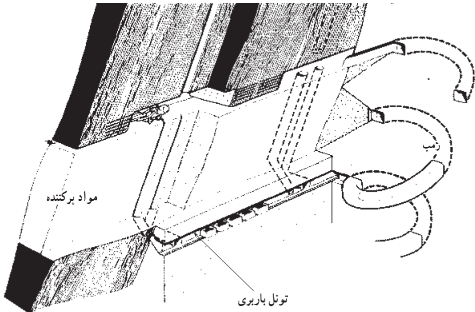
شکل ۱۰-۷- روش استخراج کردن و آکندن
