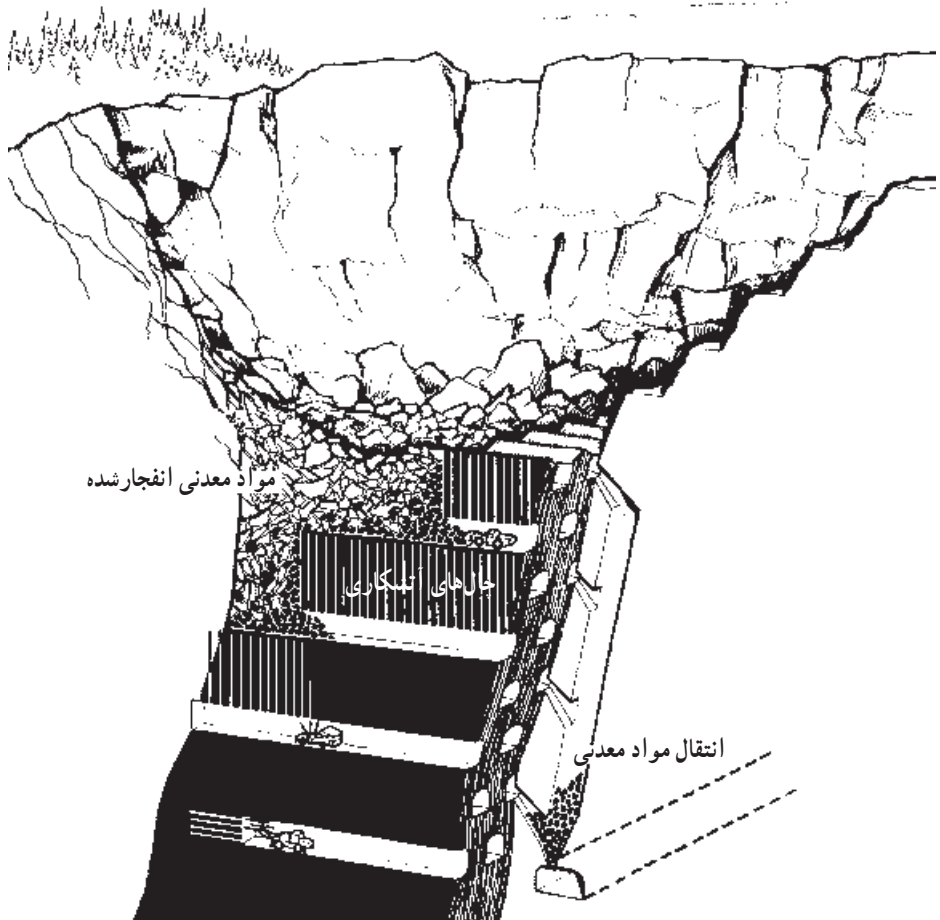
شکل ۱۶-۷- روش استخراج تخریب در طبقات فرعی
