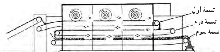
خشک‌کن‌های چندتسمه‌ای
