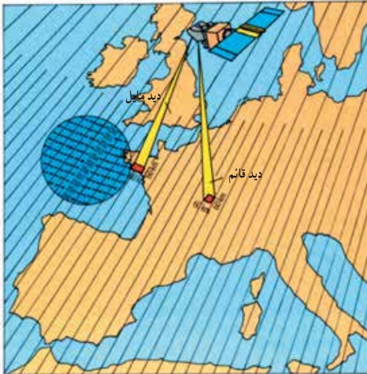
شکل ۴-۷- انواع دید ماهواره
