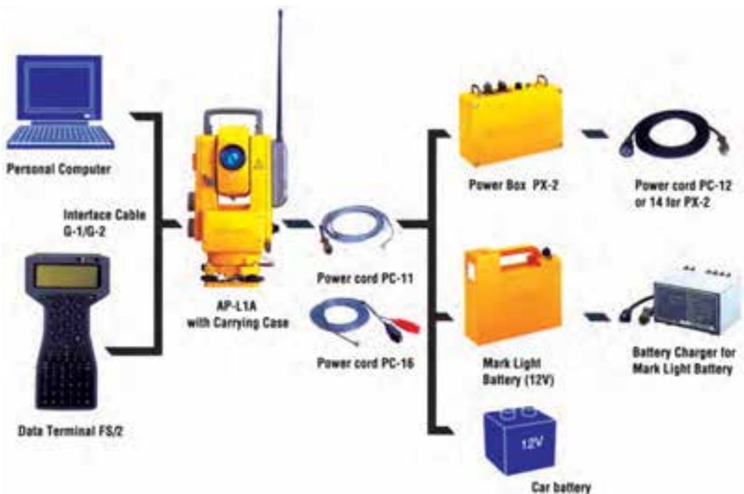
شکل ۲۲-۴- نمایش ارتباط توتال استیشن با تجهیزات جانبی
